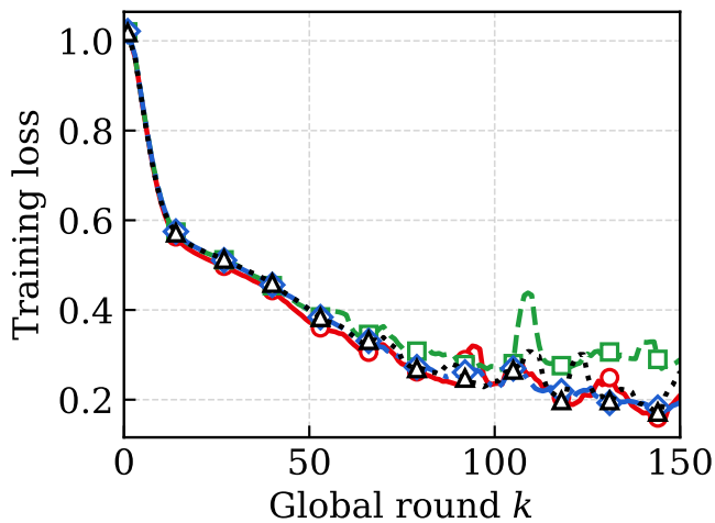
(b) nuScenes
