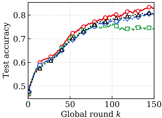
(d) nuScenes
