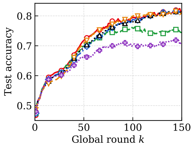
(d) nuScenes
