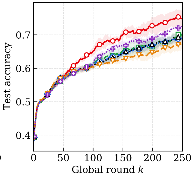
(b) nuScenes
