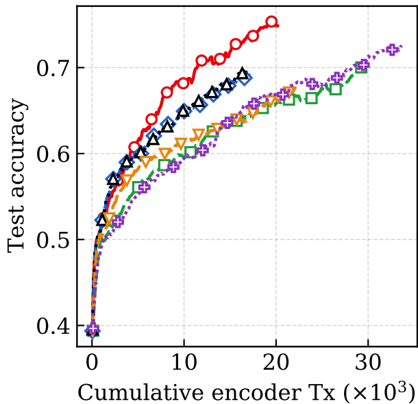
(b) nuScenes
