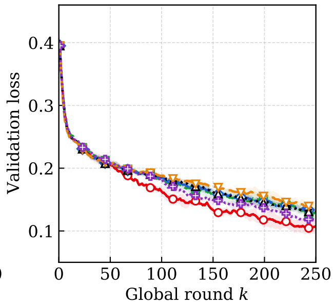
(b) nuScenes
