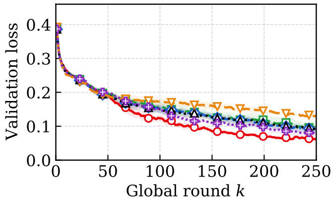
(b) nuScenes
