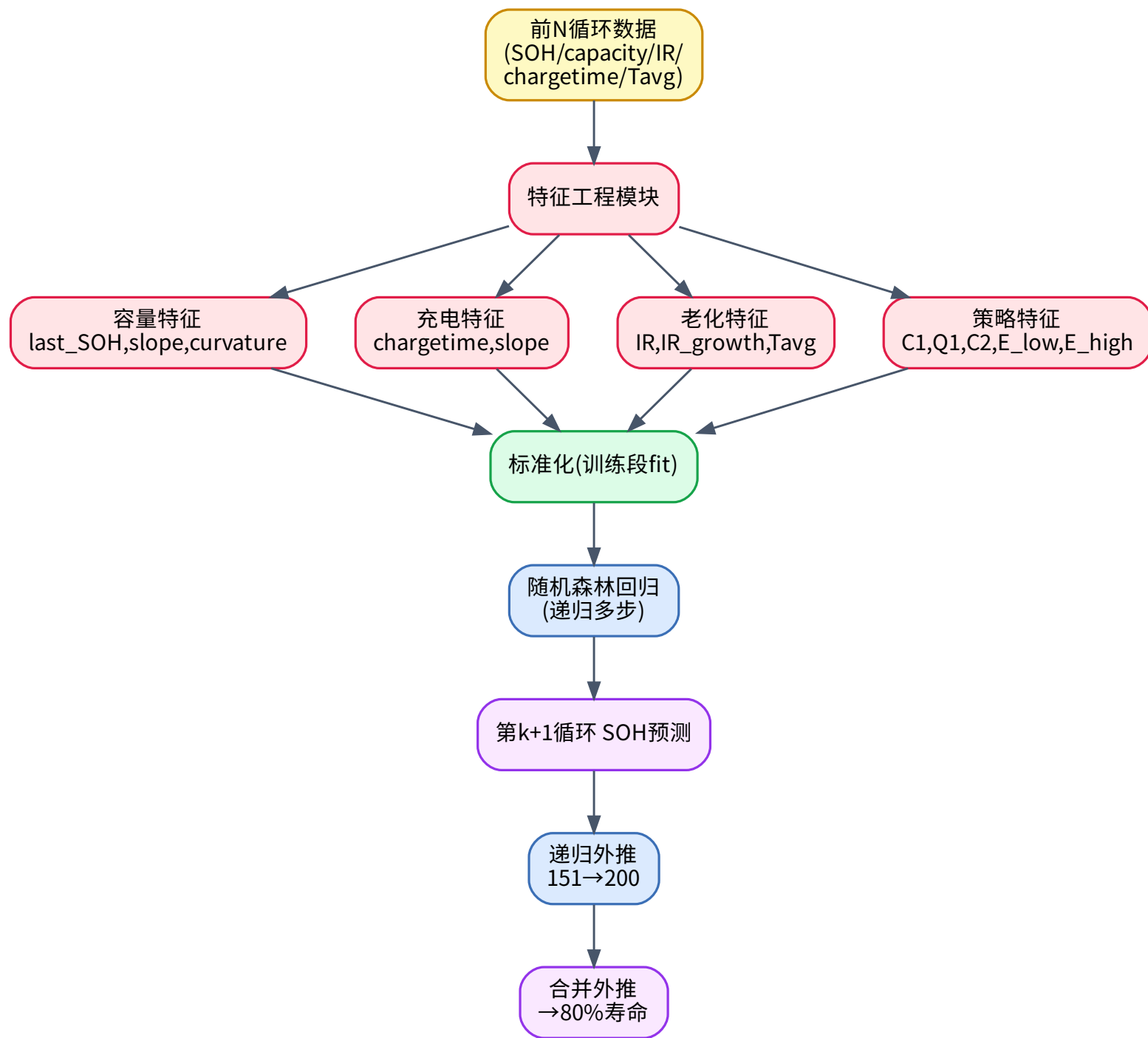
图7 问题三预测模型结构图
