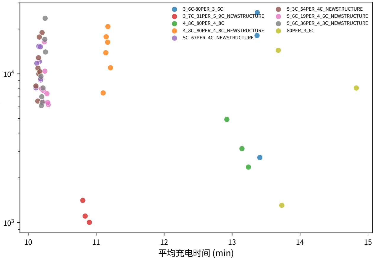
循环寿命
