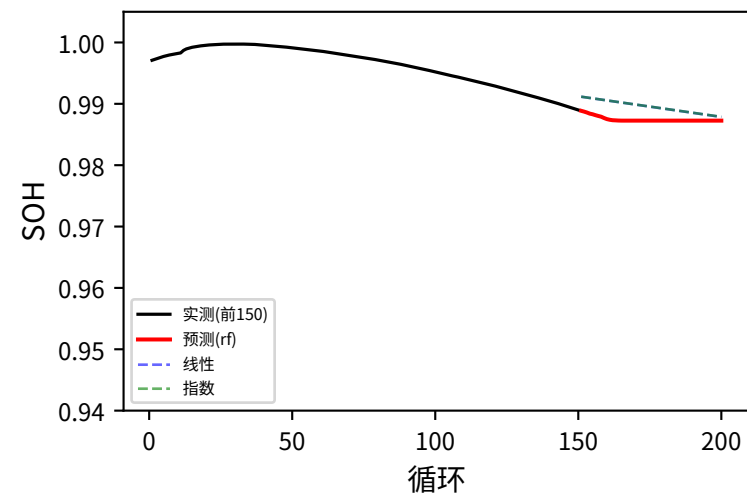
#14 5_6C_19PER_4_6C_NE 寿命预测=14895
