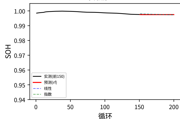
#25 4_8C_80PER_4_8C_NE 寿命预测=13117
