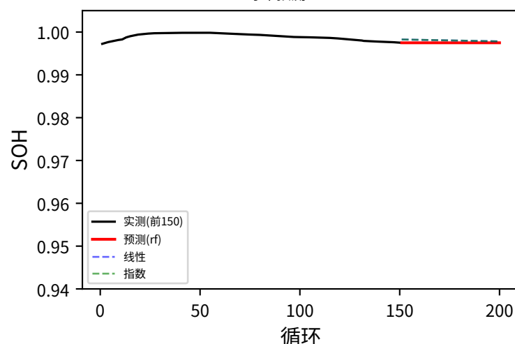
#24 5_6C_36PER_4_3C_NE 寿命预测=16770
