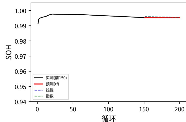
#10 5C_67PER_4C_NEWSTR 寿命预测=11200
