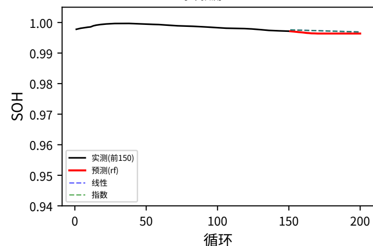
#16 3_7C_31PER_5_9C_NE 寿命预测=1330
