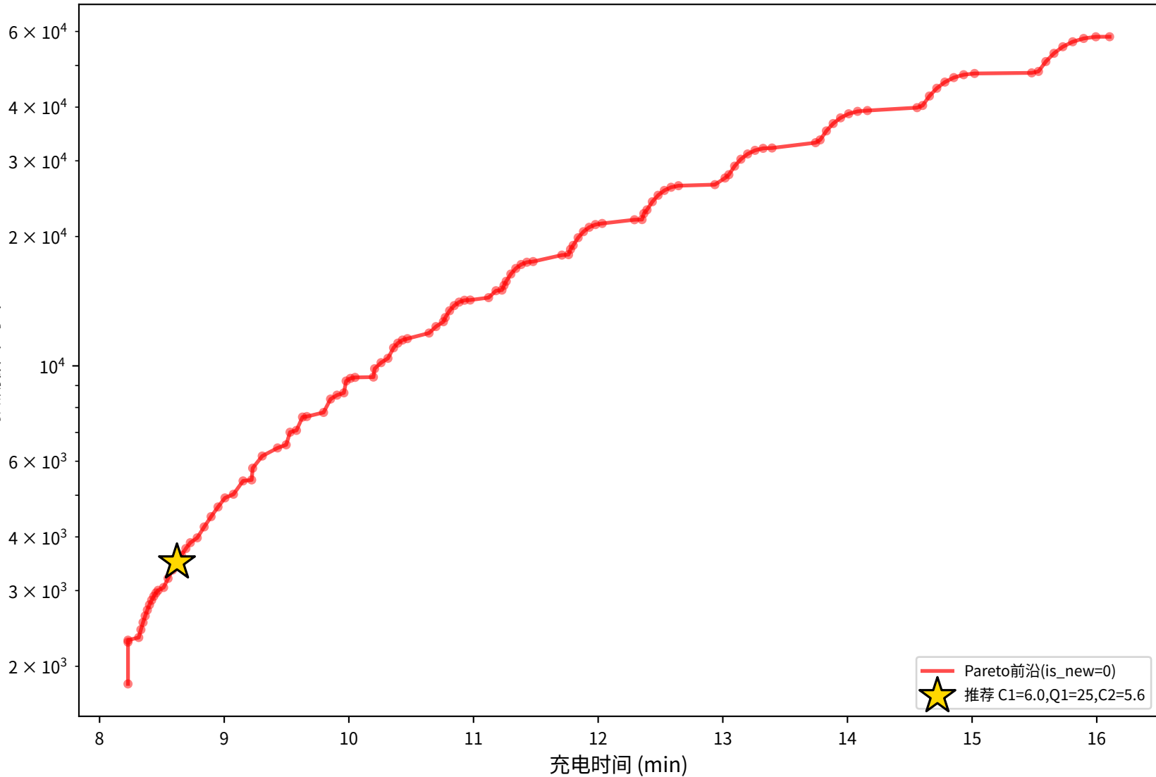
预测循环寿命
