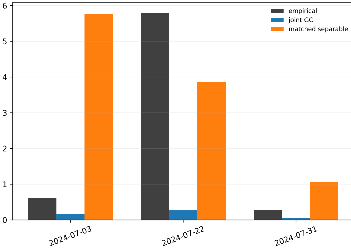
Frozen Cov(QA,QB)
