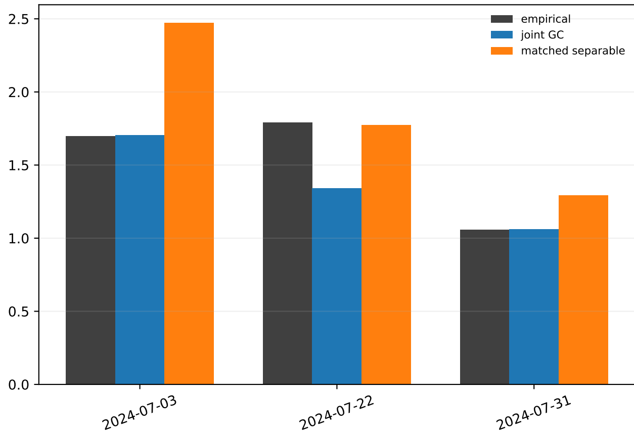
Frozen Var(L)
