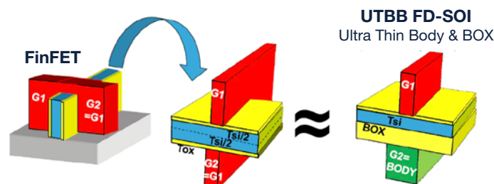
Figure 3: FinFET / FD-SOI equivalence
