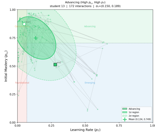
(d) Advancing ( p_{L0}, p_T ).
