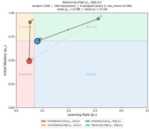
(d) Advancing (high p_{L0} , high p_T ).
