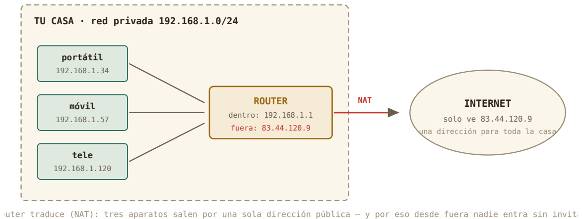
Figura 10.1: Tres aparatos dentro, una dirección fuera. El router reescribe cada paquete al salir y recuerda a quién devolver la respuesta.
