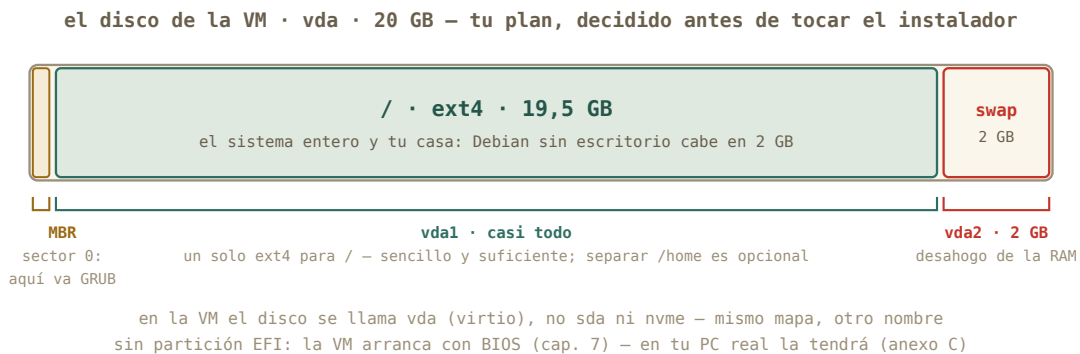
Figura 8.1: El plan de particiones para el disco virtual. Dos particiones y un sector: cada pieza con su oficio del capítulo 6.
