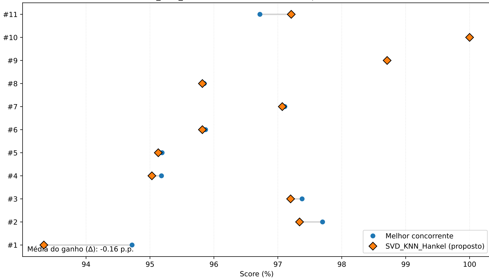
SVD_KNN_Hankel vs melhor concorrente por dataset ( \Delta )
