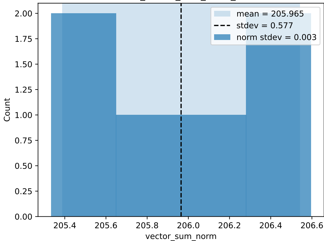
random_vector_sum_norm_stats
