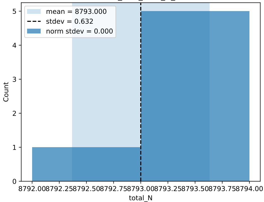
random_new_total_N_stats
