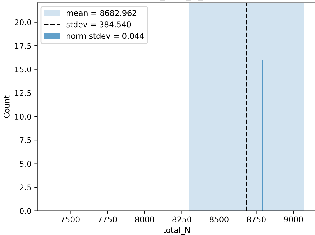
testing_total_N_stats
