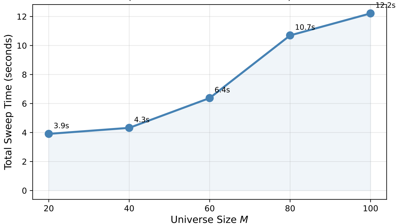
Gurobi \epsilon -Constraint Scaling ( M=20 : 3.9s \rightarrow M=100 : 3.1 \times slower)
