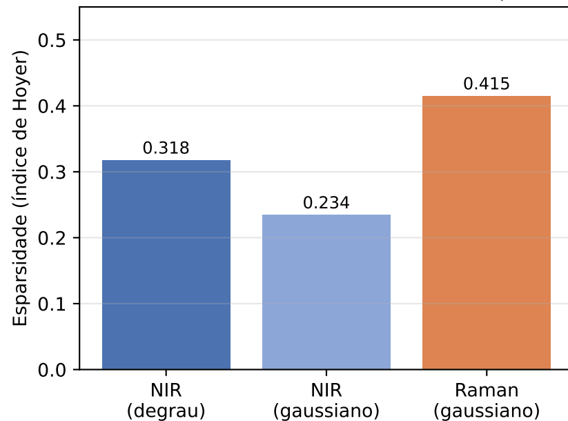
(a) H2: Esparsidade (Raman > NIR em ambas formas de prior)
