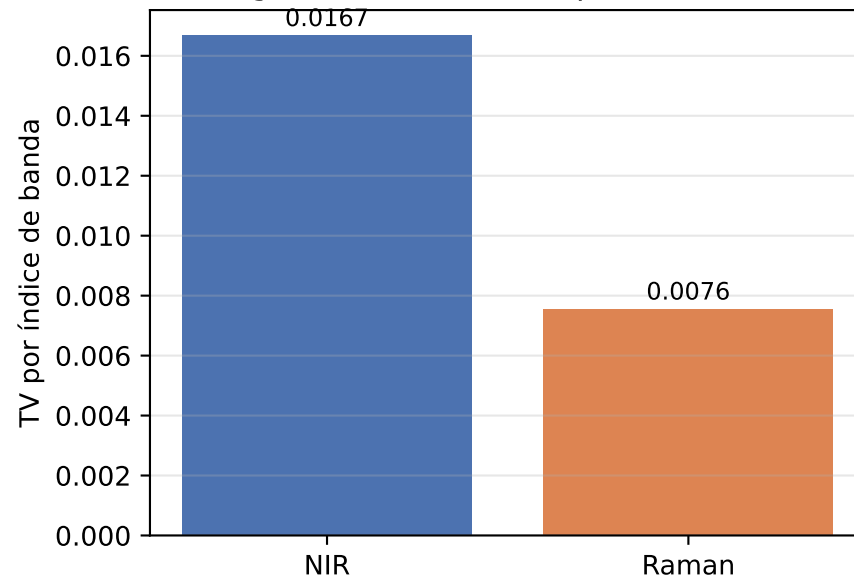
(b) Suavidade por ÍNDICE (enganosa: confundida por densidade)
