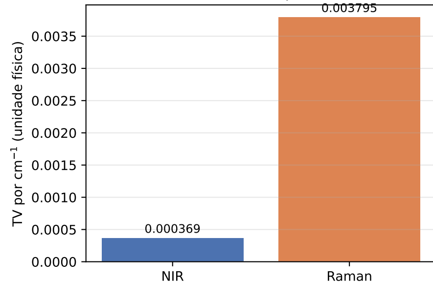
(c) H3: Suavidade FÍSICA (NIR mais suave que Raman)
