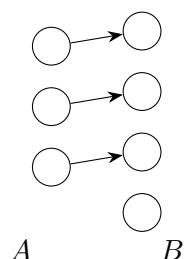
Valid function
