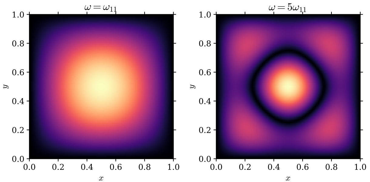
图 4.4: 同一方板在 \omega_{11} 与 5\omega_{11} 处的位移振幅。每幅图分别按其最大值归一化，因此颜色只表示模态形状，不能比较两种频率下的绝对振幅。
