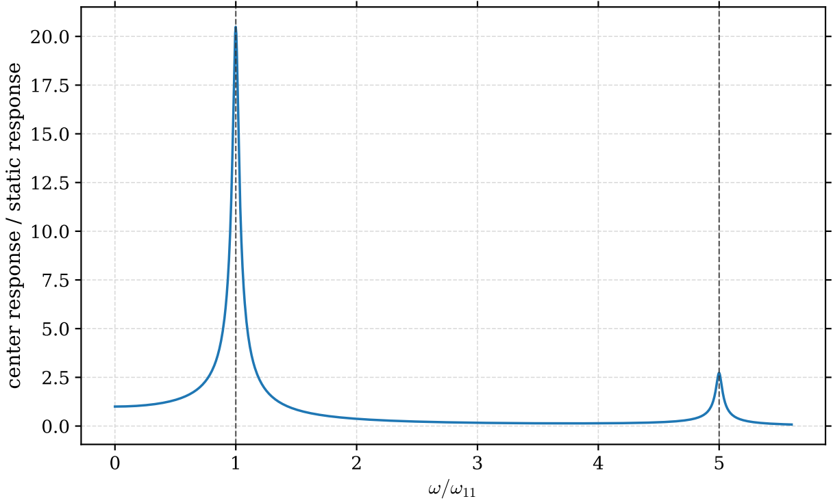
图 4.3: 均匀驱动的简支方板在轻阻尼下的中心频响。纵轴以静态中心挠度归一化；虚线标出前两个受均匀载荷激发的共振频率。
