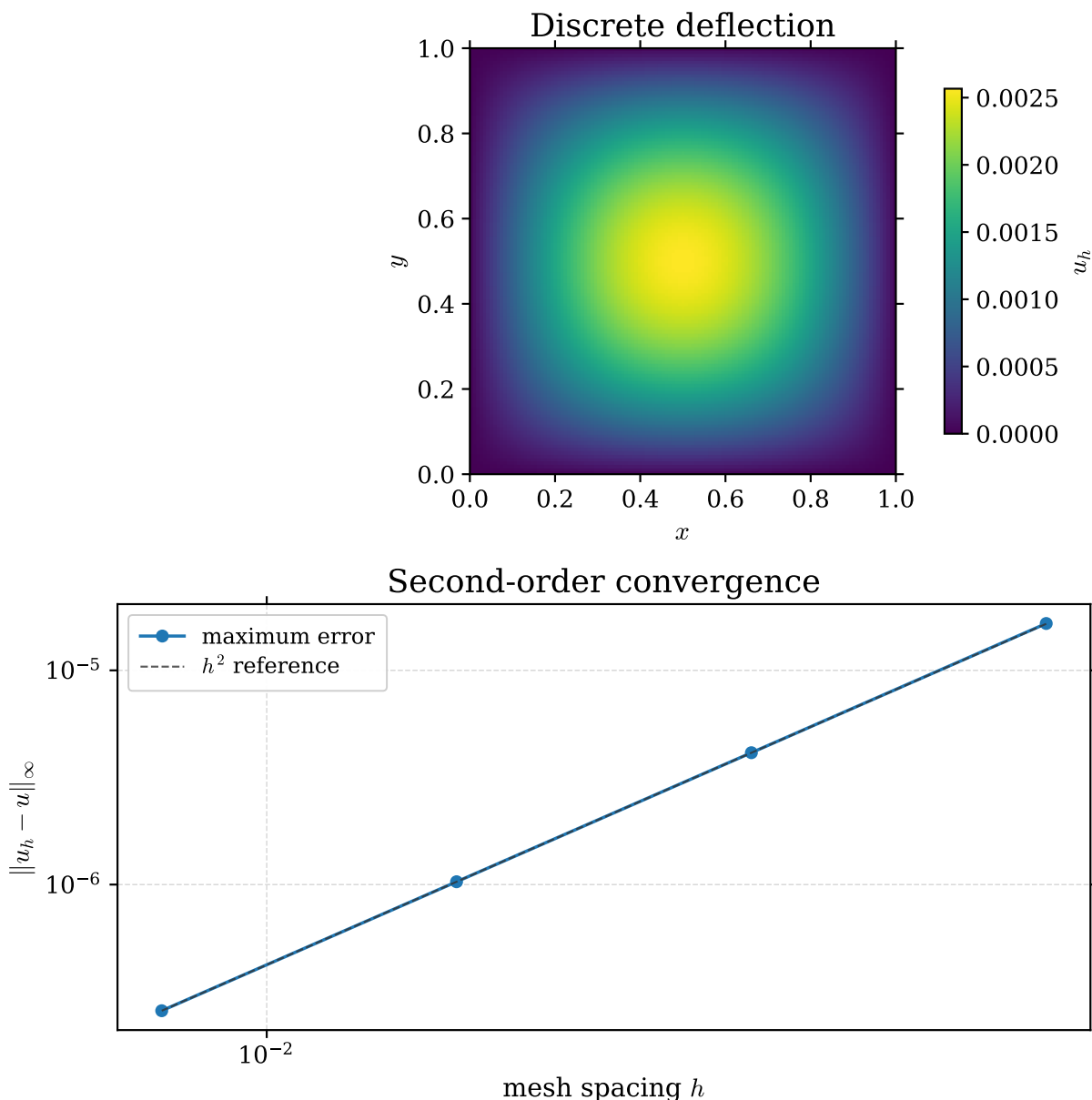
图 4.2: 单位正方形上 \Delta^2 u = \sin(\pi x) \sin(\pi y) 的 Navier 解。上图为数值挠度, 下图为相对精确式 (4.18) 的最大误差; 采用内点五点差分与两次零边界 Poisson 求解。
