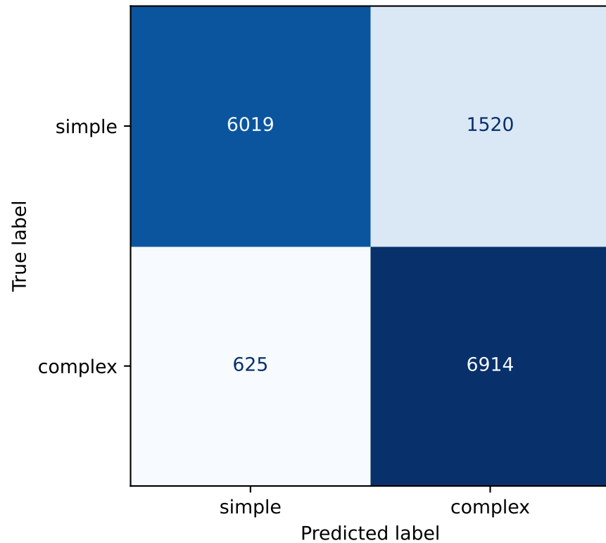
BERTino
