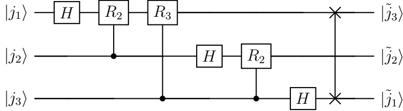
Figura 3.3: Circuito della QFT su n = 3 qubit. Ogni qubit riceve una porta di Hadamard H seguita da porte di fase controllate R_k = \text{diag}(1, e^{2\pi i/2^k}) : la rotazione applicata al qubit j dipende dai qubit successivi. Lo SWAP finale riordina i qubit nell'ordine corretto. La struttura si generalizza a n qubit richiedendo O(n^2) porte.
