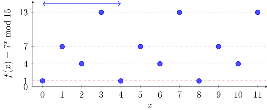
Figura 3.2: La funzione f(x) = 7^x \bmod 15 è periodica con periodo r = 4 . La periodicità è evidente dai valori che si ripetono: 1, 7, 4, 13, 1, 7, 4, 13, ... Trovare r permette di calcolare \gcd(7^2 - 1, 15) = \gcd(48, 15) = 3 e \gcd(7^2 + 1, 15) = \gcd(50, 15) = 5 , ottenendo la fattorizzazione 15 = 3 \times 5 .
