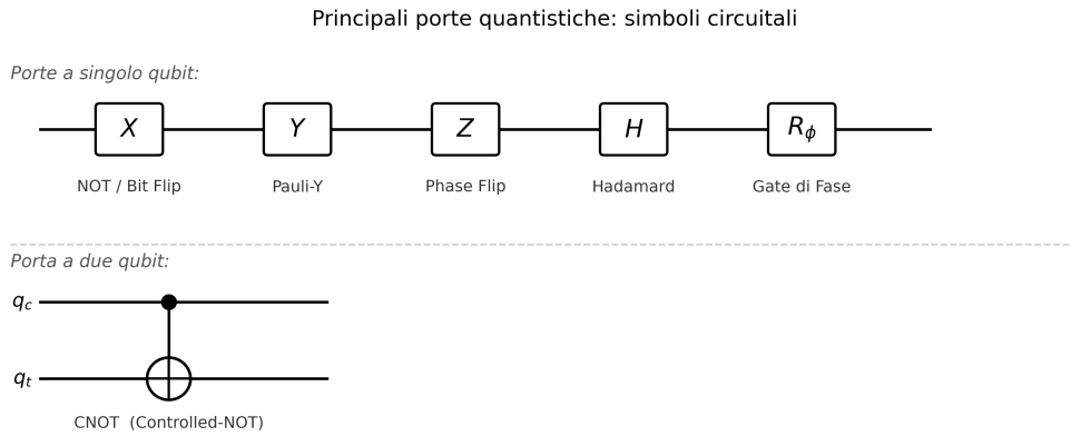
Figura B.3: Simboli circuitali delle principali porte quantistiche a singolo qubit ( X , Y , Z , H , R_\phi ) e della porta CNOT a due qubit. Nella porta CNOT, il punto pieno indica il qubit di controllo q_c e il cerchio con croce indica il qubit target q_t .
