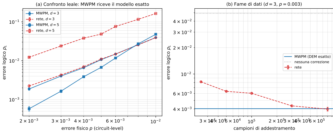
Figura 12.3: (a) Errore logico del decoder appreso e del MWPM in funzione dell'errore fisico, per d = 3 e d = 5 , con modello d'errore esatto fornito al matching. La rete affianca il matching a distanza 3 e resta al di sopra a distanza 5. (b) Errore logico della rete al crescere dell'insieme di addestramento ( d = 3 , p = 3 \times 10^{-3} ): l'avvicinamento al matching è monotono e il pareggio si raggiunge fra 3 \times 10^5 e 8 \times 10^5 campioni. Rigenerabile da figure_src/gen_qec_neural.py .
