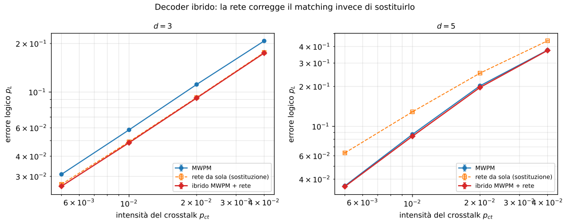
Figura 12.6: Errore logico dei tre decoder in funzione dell'intensità del crosstalk. L'ibrido (rosso) è il migliore a entrambe le distanze; la rete usata come sostituto (arancio) domina il matching a d = 3 ma lo perde a d = 5 , dove l'ibrido continua invece a guadagnare.
