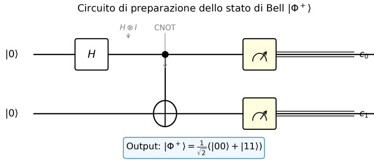
Figura B.2: Circuito quantistico per la preparazione dello stato di Bell |\Phi^+\rangle . Una porta di Hadamard H posta sul qubit di controllo crea la sovrapposizione \frac{1}{\sqrt{2}}(|0\rangle + |1\rangle) ; la successiva porta CNOT introduce le correlazioni di entanglement, producendo lo stato \frac{1}{\sqrt{2}}(|00\rangle + |11\rangle) .
