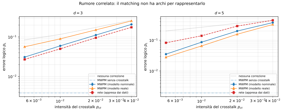
Figura 12.4: Errore logico in funzione dell'intensità del crosstalk, a errore fisico costante p = 3 \times 10^{-3} . A distanza 3 la rete (rosso) domina il matching sia con modello nominale (blu) sia con modello reale (arancio), che risulta il peggiore; a distanza 5 l'ordine si inverte. La linea tratteggiata inferiore indica l'errore logico del matching in assenza di crosstalk, cioè il livello che la decodifica raggiungerebbe se il modello fosse corretto.
