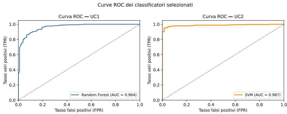
Figura F.1: Curve ROC dei classificatori selezionati: Random Forest per UC1 (AUC=0.964) e SVM per UC2 (AUC=0.987). La linea tratteggiata rappresenta il classificatore casuale (AUC=0.5).
