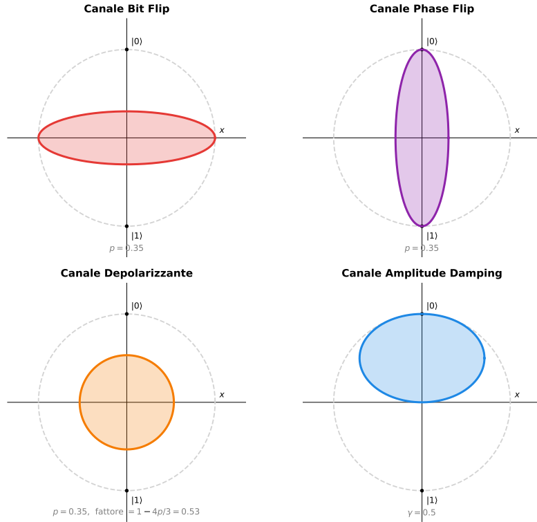
Figura 5.5: Effetto dei quattro canali di rumore sulla sfera di Bloch (sezione nel piano xz ). La curva tratteggiata grigia rappresenta la sfera ideale; la superficie colorata è la sfera dopo l'applicazione del canale con il parametro indicato. Il Bit Flip contrae la sfera lungo z ; il Phase Flip lungo x (distrugge le coerenze equatoriali); il canale Depolarizzante contrae isotropicamente verso il centro; l'Amplitude Damping sposta la sfera verso il polo nord |0\rangle .
