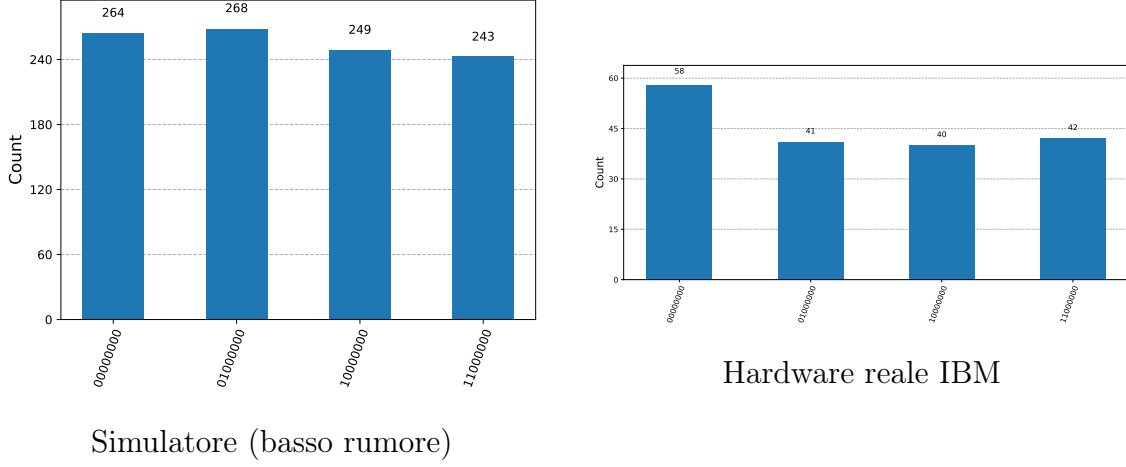
Figura 14.1: Confronto degli istogrammi QPE per N = 15 con base a = 2 su simulatore (sinistra) e su hardware IBM Quantum reale (destra). Entrambi gli istogrammi provengono dall'esecuzione del notebook del tutorial ufficiale IBM [4] sul processore ibm_marrakesh , e non dalla pipeline sperimentale di questa tesi, che opera su simulatore e adotta la base a = 7 (Capitolo 10): sono riportati qui come termine di paragone qualitativo, non come misura propria. Sul simulatore i quattro picchi corretti \{0, 64, 128, 192\} raccolgono \approx 250 conteggi ciascuno su 1024 shot; sull'hardware reale gli stessi picchi risultano significativamente più deboli ( \approx 40 – 58 conteggi), con la maggior parte dei conteggi dispersi uniformemente. Il divario dà la misura qualitativa della distanza fra un modello di rumore statico e il rumore reale, correlato e non stazionario, di un processore fisico.
