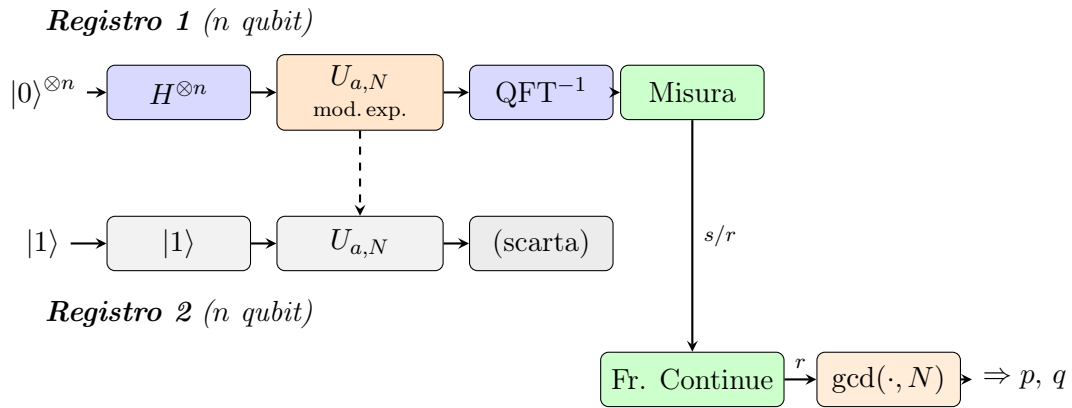
Figura 4.7: Schema a due registri dell'algoritmo di Shor. Il Registro 1 (di controllo) viene posto in sovrapposizione uniforme con H^{\otimes n} , entangled con il Registro 2 tramite la moltiplicazione modulare U_{a,N} , quindi trasformato con la \text{QFT}^{-1} . La misura produce un valore s/r elaborato classicamente: le frazioni continue stimano il periodo r , e il calcolo del MCD restituisce i fattori p e q di N .
