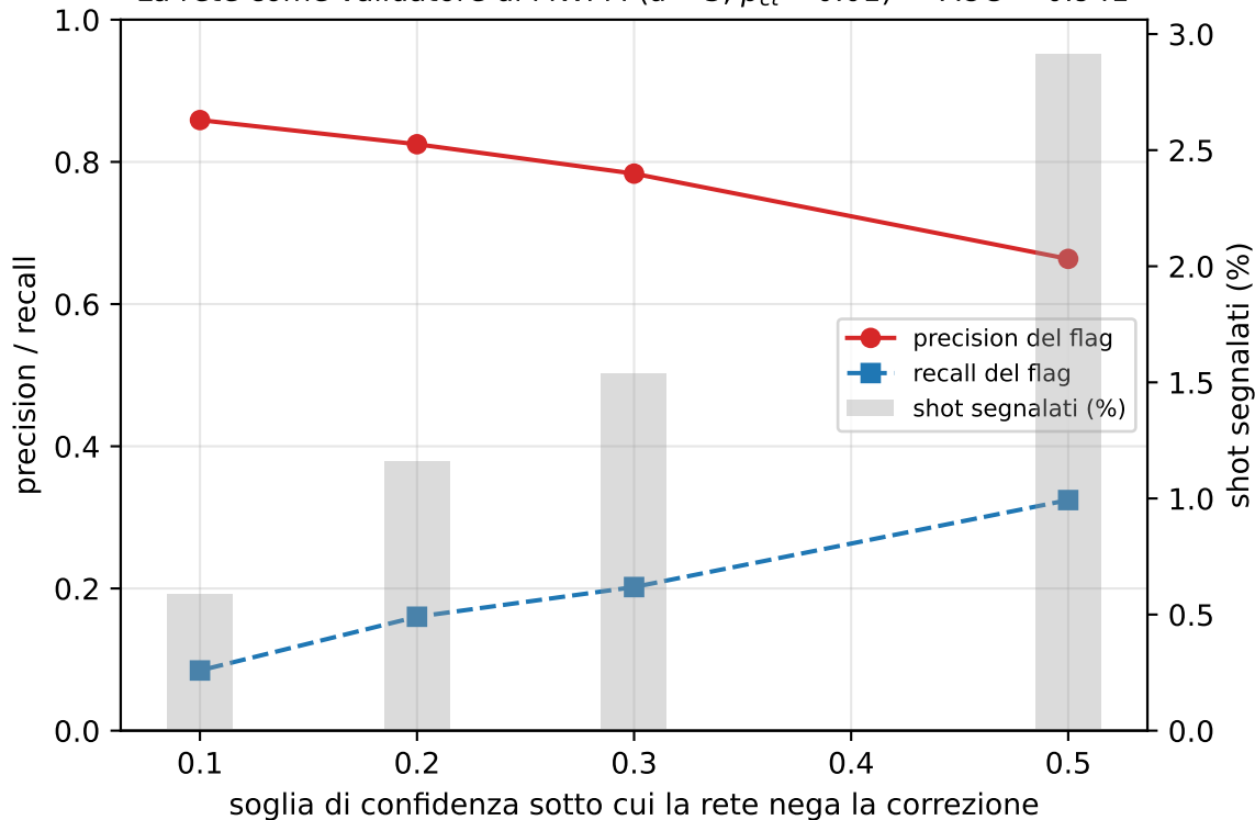
La rete come validatore di MWPM ( d = 3 , p_{ct} = 0.01 ) — AUC = 0.941
