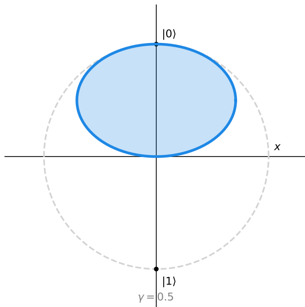
Canale Amplitude Damping
