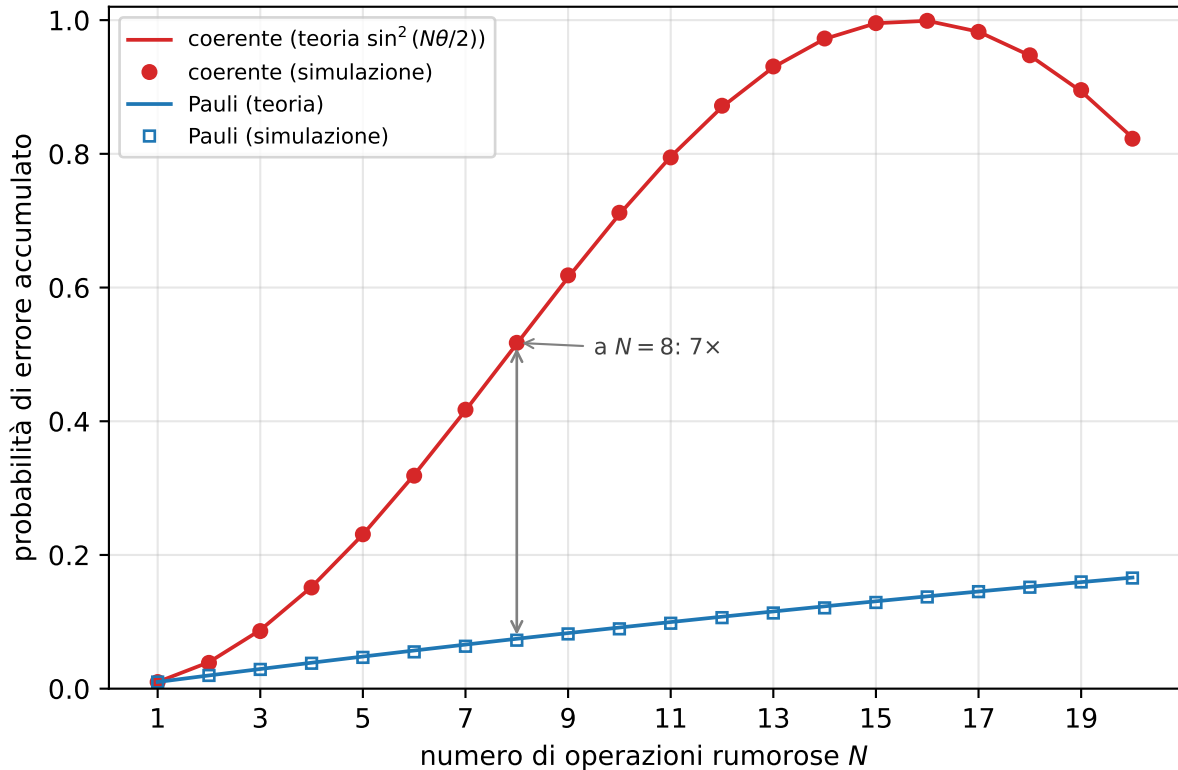
Errori coerenti vs Pauli (stessa p = 0.01 per operazione)
