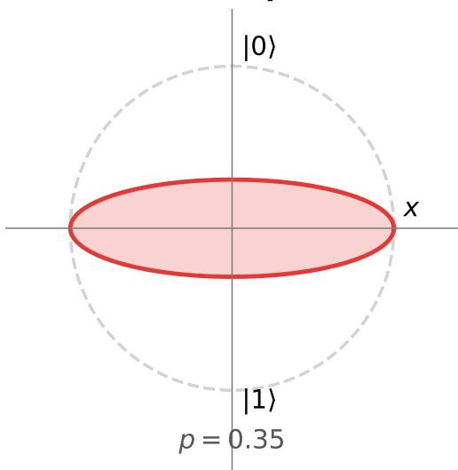
Depolarizzante
