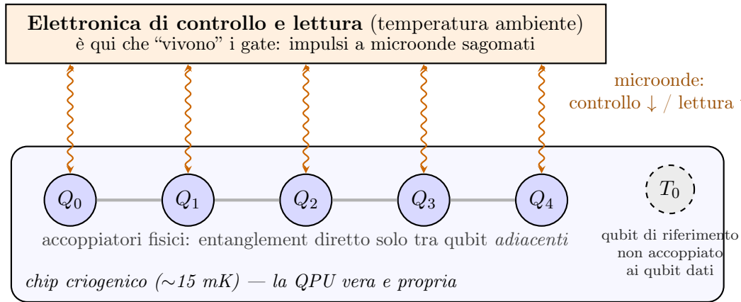
Figura A.3: Schema didattico di una QPU superconduttiva: cinque qubit in catena, qubit di riferimento T_0 ed elettronica esterna di controllo e lettura.
