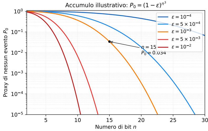
Figura A.6: Proxy illustrativo (1 - \epsilon)^{n^3} per cinque valori di \epsilon . La curva non deriva dai circuiti sperimentali e mostra soltanto l'accumulo moltiplicativo di eventi.
