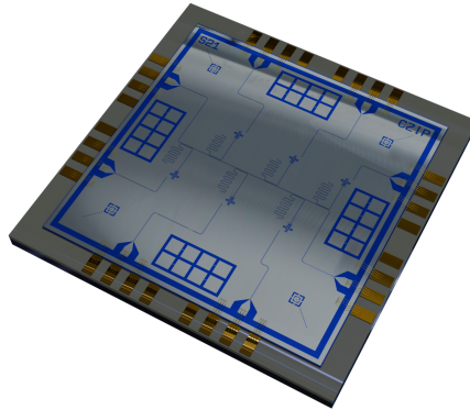
Figura A.5: Resa tridimensionale di un chip a sei transmon e dodici giunzioni di test. Credito: Onri Jay Benally, CC BY 4.0, via Wikimedia Commons.
