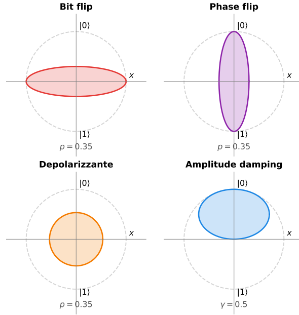
Figura A.7: Effetto dei quattro canali nel piano xz . La curva tratteggiata è la sfera ideale: bit flip e phase flip contraggono direzioni selettive, il depolarizzante contrae isotropicamente e l'amplitude damping sposta lo stato verso |0\rangle .
