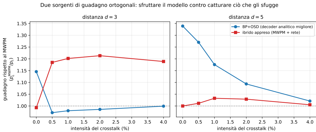
Figura E.2: Guadagno di BP+OSD (blu) e del decoder ibrido (rosso) rispetto al MWPM, al variare del crosstalk. La linea tratteggiata indica il guadagno unitario; i pannelli distinguono le distanze 3 e 5.
