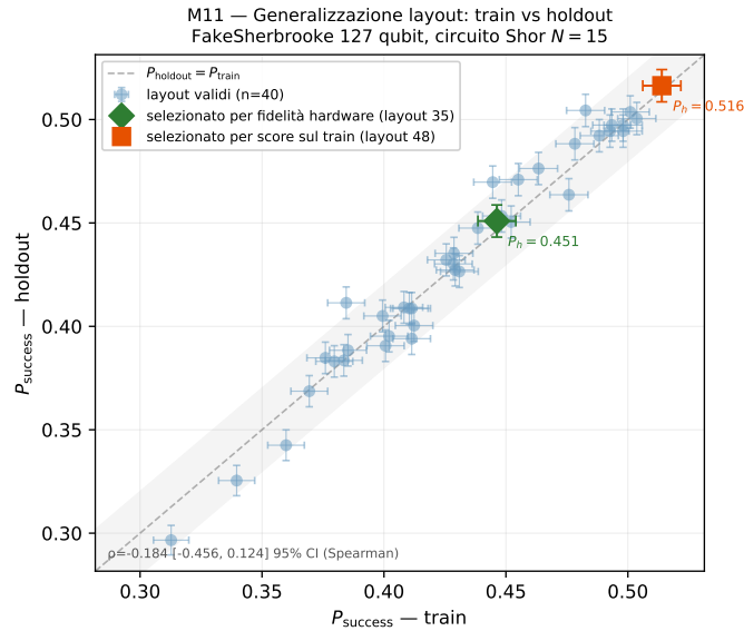
Figura E.3: Successo in selezione e in holdout dei 40 layout M11, con barre di errore e diagonale y = x . Sono evidenziati i layout scelti dal punteggio di calibrazione (ID 35) e dal successo in selezione (ID 48).
