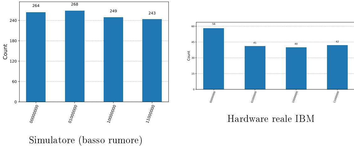
Figura 11.1: Confronto degli istogrammi QPE per N = 15 , a = 7 su simulatore (sinistra) e su hardware IBM Quantum reale (destra). Sul simulatore i quattro picchi corretti \{0, 64, 128, 192\} raccolgono \approx 250 conteggi ciascuno su 1024 shot; sull'hardware reale gli stessi picchi risultano significativamente più deboli ( \approx 40 – 58 conteggi), con la maggior parte dei conteggi dispersi uniformemente. Questo simulation gap quantifica la distanza tra il modello di rumore statico adottato e il rumore reale correlato e non stazionario del processore fisico.
