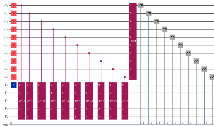
Figura 10.1: Circuito di Quantum Phase Estimation per N = 21 , a = 2 ( n_{\text{count}} = 10 qubit di controllo, 5 qubit target). La struttura è analoga a N = 15 ma con un registro di controllo più ampio e blocchi di moltiplicazione modulare controllata ( M_2, M_4, M_{16}, \dots ) più profondi. La complessità risultante con decomposizione UnitaryGate porta a 10 040 porte CX dopo la traspilazione.
