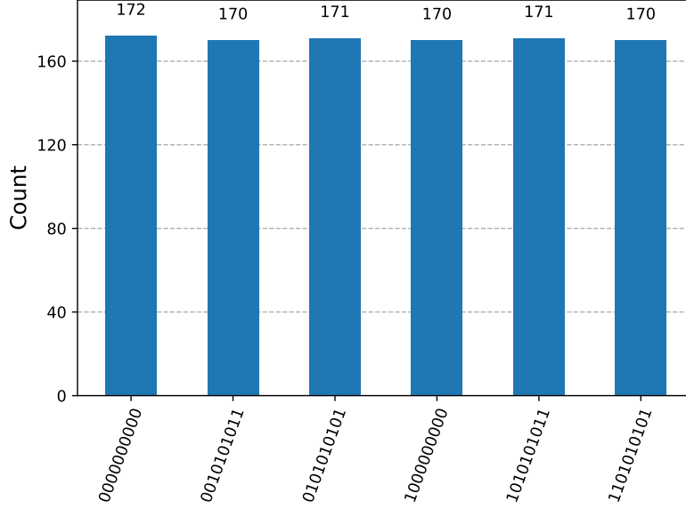
Figura 10.2: Distribuzione di misura del registro di controllo per N = 21 con decomposizione UnitaryGate (1024 shot, noise model NISQ-realistico). I sei stati più frequenti hanno conteggi pressoché identici ( \approx 170 ciascuno): l'output è indistinguibile da una distribuzione uniforme, confermando che P_{\text{surv}} \approx 10^{-44} annulla qualsiasi segnale QPE.
