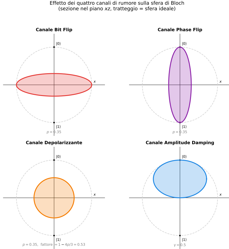
Figura 5.1: Effetto dei quattro canali di rumore sulla sfera di Bloch (sezione nel piano xz ). La curva tratteggiata grigia rappresenta la sfera ideale; la superficie colorata è la sfera dopo l'applicazione del canale con il parametro indicato. Il Bit Flip contrae la sfera lungo z ; il Phase Flip lungo x (distrugge le coerenze equatoriali); il canale Depolarizzante contrae isotropicamente verso il centro; l'Amplitude Damping sposta la sfera verso il polo nord |0\rangle .
