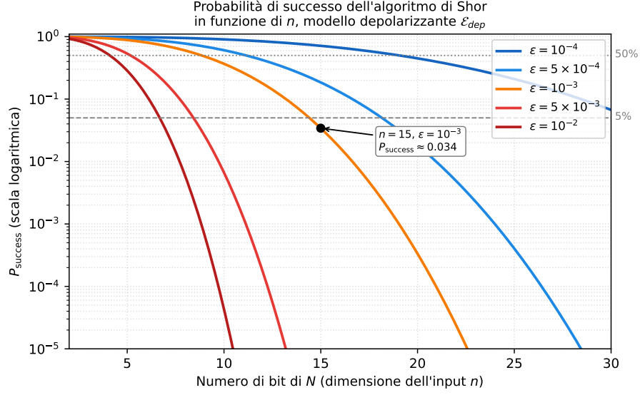
Figura 5.2: Probabilità di successo dell'algoritmo di Shor P_{\text{success}} \approx (1 - \epsilon)^{n^3} in funzione della dimensione dell'input n (in bit), per cinque valori di intensità di rumore depolarizzante \epsilon . Anche con \epsilon = 10^{-3} (fedeltà gate 99.9%), già per n = 15 la probabilità di ottenere un risultato corretto scende al 3.4%. Le linee tratteggiate orizzontali evidenziano le soglie del 50% e del 5%.
