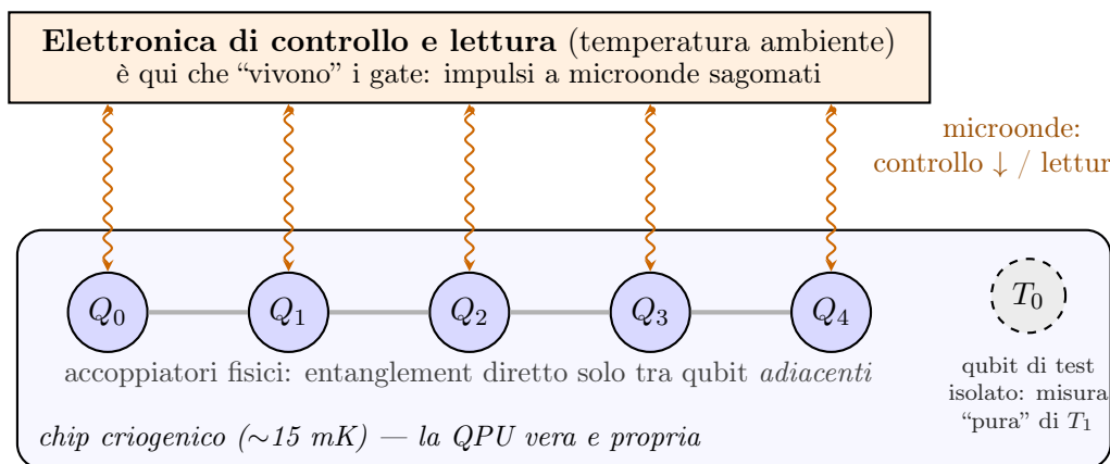
Figura 5.1: Anatomia di una QPU superconduttiva a 5 qubit con topologia a catena lineare. Nel chip criogenico risiedono solo i qubit e gli accoppiatori fisici; le porte logiche sono impulsi a microonde generati dall'elettronica esterna e convogliati tramite guide d'onda, usate sia per il controllo sia per la lettura. L'entanglement diretto è possibile solo tra qubit adiacenti ( Q_1 – Q_2 sì, Q_0 – Q_2 solo tramite operazioni intermedie, che amplificano il disturbo). Il qubit di test T_0 , privo di collegamenti, serve a misurare il tempo di coerenza “puro”: un qubit collegato a una guida d'onda perde sempre un po' di energia attraverso di essa.
