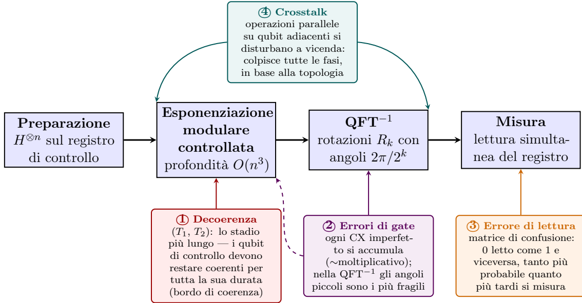
Figura 5.2: Localizzazione delle quattro fonti fisiche di rumore sulla pipeline dell’algoritmo di Shor. La decoerenza ① domina l’esponenziazione modulare (lo stadio più profondo, O(n^3) gate); gli errori di gate ② si accumulano su tutti i CX e sono particolarmente critici sulle rotazioni ad angolo piccolo della QFT^{-1} ; l’errore di lettura ③ colpisce la misura finale, tanto più quanto più il circuito arriva “lungo” al bordo di coerenza; il crosstalk ④ agisce trasversalmente ovunque vi siano operazioni parallele su qubit adiacenti, secondo la topologia del dispositivo (Sezione 5.2).
