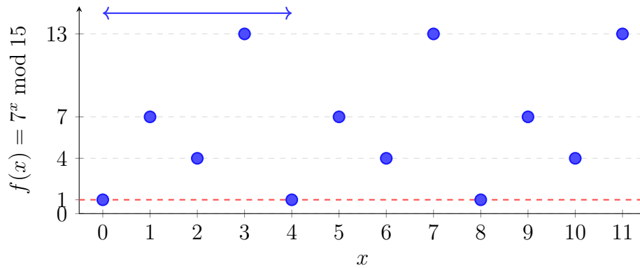
Figura 4.1: La funzione f(x) = 7^x \bmod 15 è periodica con periodo r = 4 . La periodicità è evidente dai valori che si ripetono: 1, 7, 4, 13, 1, 7, 4, 13, \dots . Trovare r permette di calcolare \gcd(7^2 - 1, 15) = \gcd(48, 15) = 3 e \gcd(7^2 + 1, 15) = \gcd(50, 15) = 5 , ottenendo la fattorizzazione 15 = 3 \times 5 .
