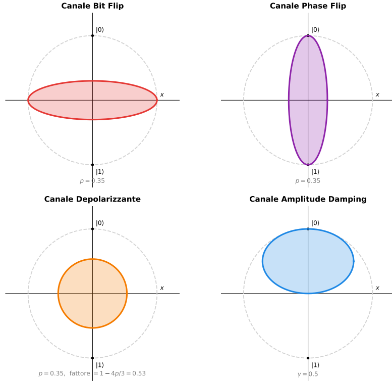
Figura 5.1: Effetto dei quattro canali di rumore sulla sfera di Bloch (sezione nel piano xz ). La curva tratteggiata grigia rappresenta la sfera ideale; la superficie colorata è la sfera dopo l'applicazione del canale con il parametro indicato. Il Bit Flip contrae la sfera lungo z ; il Phase Flip lungo x (distrugge le coerenze equatoriali); il canale Depolarizzante contrae isotropicamente verso il centro; l'Amplitude Damping sposta la sfera verso il polo nord |0\rangle .
