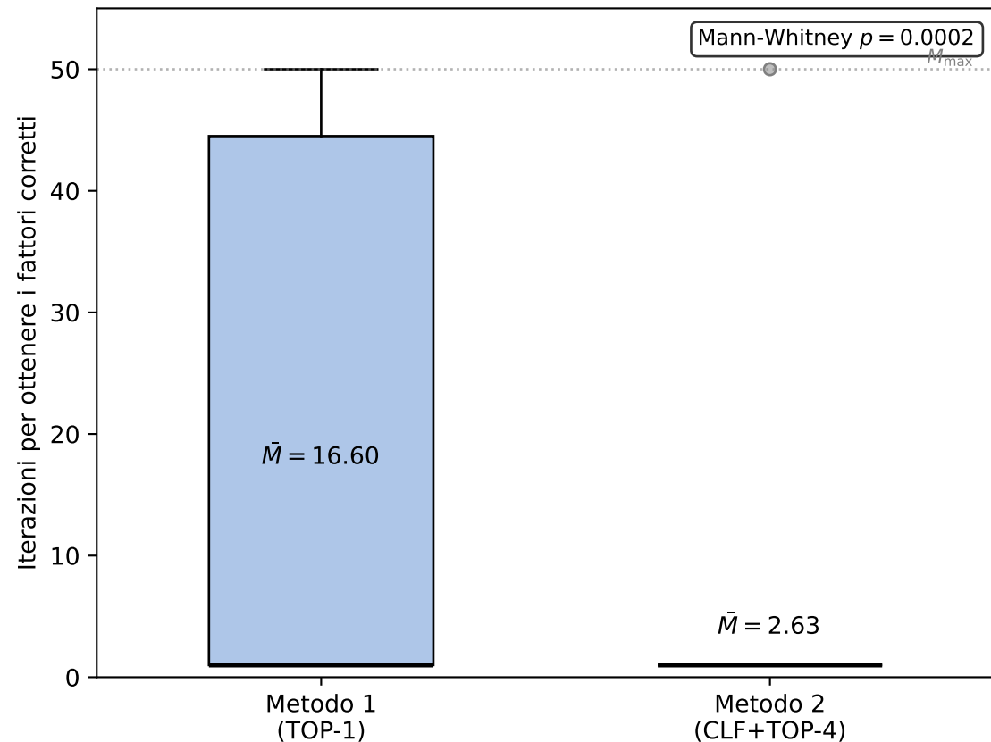
UC1 — Distribuzione iterazioni: Metodo 1 vs Metodo 2 ( N = 15 , NISQ-realistico, K = 30 ripetizioni, M_{\max} = 50 )
