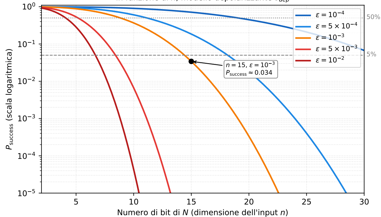
Probabilità di successo dell' algoritmo di Shor in funzione di n , modello depolarizzante \mathcal{E}_{dep}
