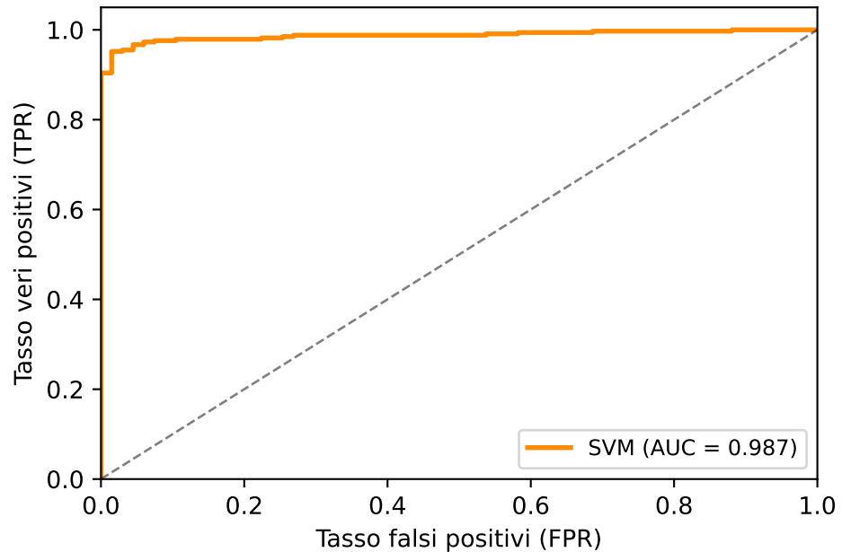
Curva ROC — UC2
