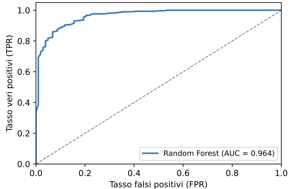
Curva ROC — UC1
