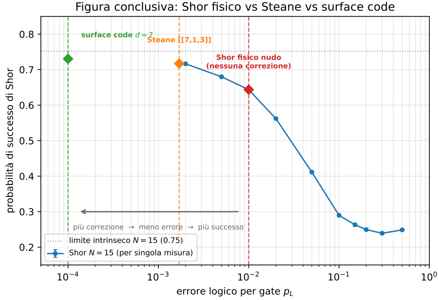
Figura 13.1: Probabilità di successo di Shor ( N = 15 ) in funzione dell'errore logico per gate p_L . La curva scende in modo monotono dal limite intrinseco dell'istanza (0.75 a p_L \rightarrow 0 ) fino al livello di successo casuale ( \approx 0.25 ). I tre marcatori collocano i regimi di correzione (errore logico residuo dai Capitoli 11 e 12): Shor fisico nudo ( p_L \approx 10^{-2} , nessuna correzione), codice di Steane ( p_L \approx 1.7 \times 10^{-3} ) e surface code d = 7 ( p_L \approx 10^{-4} ). Muovendosi verso sinistra — cioè aumentando la capacità di correzione — l'errore logico cala e P_{\text{success}} risale verso il limite. Curva rigenerabile da figure_src/gen_shor_logico.py .
