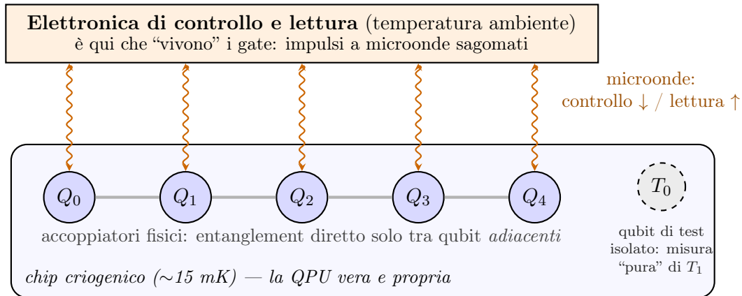
Figura A.4: Anatomia di una QPU superconduttiva a 5 qubit con topologia a catena lineare. Nel chip criogenico risiedono solo i qubit e gli accoppiatori fisici; le porte logiche sono impulsi a microonde generati dall’elettronica esterna e convogliati tramite guide d’onda, usate sia per il controllo sia per la lettura. L’entanglement diretto è possibile solo tra qubit adiacenti ( Q_1 – Q_2 sì, Q_0 – Q_2 solo tramite operazioni intermedie, che amplificano il disturbo). Il qubit di test T_0 , privo di collegamenti, serve a misurare il tempo di coerenza “puro”: un qubit collegato a una guida d’onda perde sempre un po’ di energia attraverso di essa.
