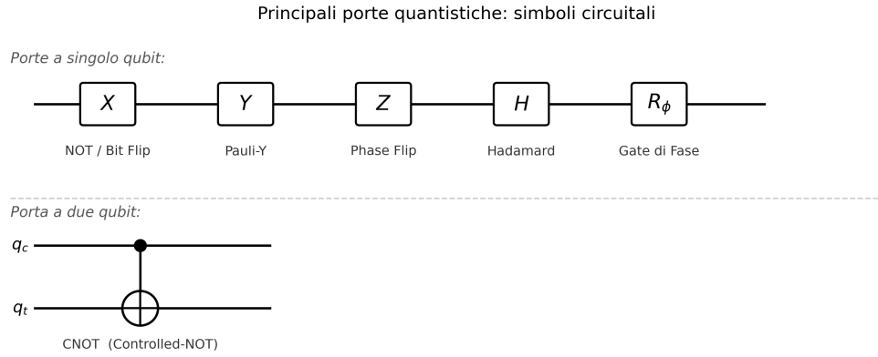
Figura A.2: Simboli circuitali delle principali porte quantistiche a singolo qubit ( X , Y , Z , H , R_\phi ) e della porta CNOT a due qubit. Nella porta CNOT, il punto pieno indica il qubit di controllo q_c e il cerchio con croce indica il qubit target q_t .
