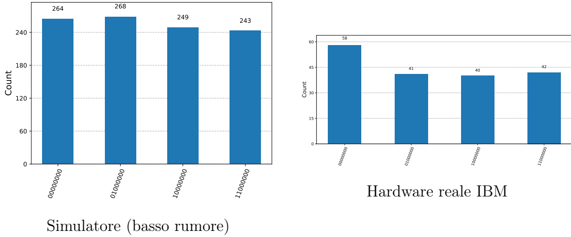
Figura 11.1: Confronto degli istogrammi QPE per N = 15 con base a = 2 su simulatore (sinistra) e su hardware IBM Quantum reale (destra). Entrambi gli istogrammi provengono dall'esecuzione del notebook del tutorial ufficiale IBM [4] sul processore ibm_marrakesh , e non dalla pipeline sperimentale di questa tesi, che opera su simulatore e adotta la base a = 7 (Capitolo 7): sono riportati qui come termine di paragone qualitativo, non come misura propria. Sul simulatore i quattro picchi corretti \{0, 64, 128, 192\} raccolgono \approx 250 conteggi ciascuno su 1024 shot; sull'hardware reale gli stessi picchi risultano significativamente più deboli ( \approx 40 – 58 conteggi), con la maggior parte dei conteggi dispersi uniformemente. Il divario dà la misura qualitativa della distanza fra un modello di rumore statico e il rumore reale, correlato e non stazionario, di un processore fisico.
