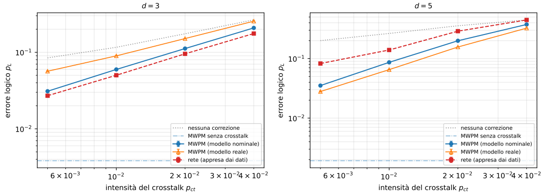
Figura 12.4: Errore logico in funzione dell'intensità del crosstalk, a errore fisico costante p = 3 \times 10^{-3} . A distanza 3 la rete (rosso) domina il matching sia con modello nominale (blu) sia con modello reale (arancio), che risulta il peggiore; a distanza 5 l'ordine si inverte. La linea tratteggiata inferiore indica l'errore logico del matching in assenza di crosstalk, cioè il livello che la decodifica raggiungerebbe se il modello fosse corretto.
