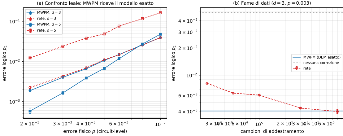
Figura 12.3: (a) Errore logico del decoder appreso e del MWPM in funzione dell'errore fisico, per d = 3 e d = 5 , con modello d'errore esatto fornito al matching. La rete affianca il matching a distanza 3 e resta al di sopra a distanza 5. (b) Errore logico della rete al crescere dell'insieme di addestramento ( d = 3, p = 3 \times 10^{-3} ): l'avvicinamento al matching è monotono e il pareggio si raggiunge fra 3 \times 10^5 e 8 \times 10^5 campioni. Rigenerabile da figure_src/gen_qec_neural.py .
