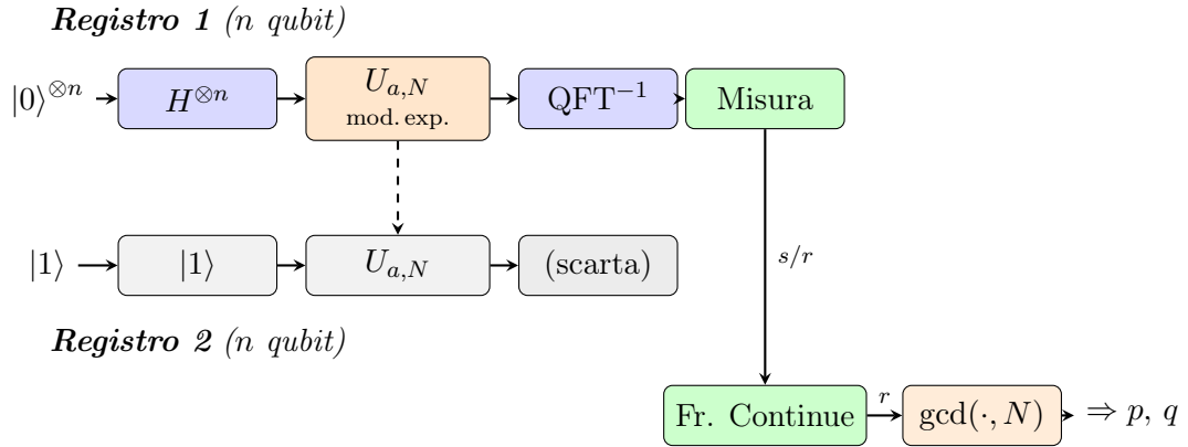
Figura 4.7: Schema a due registri dell'algoritmo di Shor. Il Registro 1 (di controllo) viene posto in sovrapposizione uniforme con H^{\otimes n} , entangled con il Registro 2 tramite la moltiplicazione modulare U_{a,N} , quindi trasformato con la \text{QFT}^{-1} . La misura produce un valore s/r elaborato classicamente: le frazioni continue stimano il periodo r , e il calcolo del MCD restituisce i fattori p e q di N .
