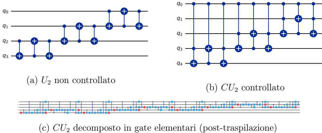
Figura 4.4: Gate di moltiplicazione modulare U_2 |x\rangle = |2x \bmod 15\rangle per N = 15 , a = 2 . (a) Versione non controllata su 4 qubit: implementata come sequenza di SWAP. (b) Versione controllata CU_2 su 5 qubit utilizzata nel circuito QPE. (c) Decomposizione in gate elementari dopo la traspilazione: le porte SWAP si espandono in triple di CNOT, rivelando il costo effettivo in gate a due qubit del blocco.
