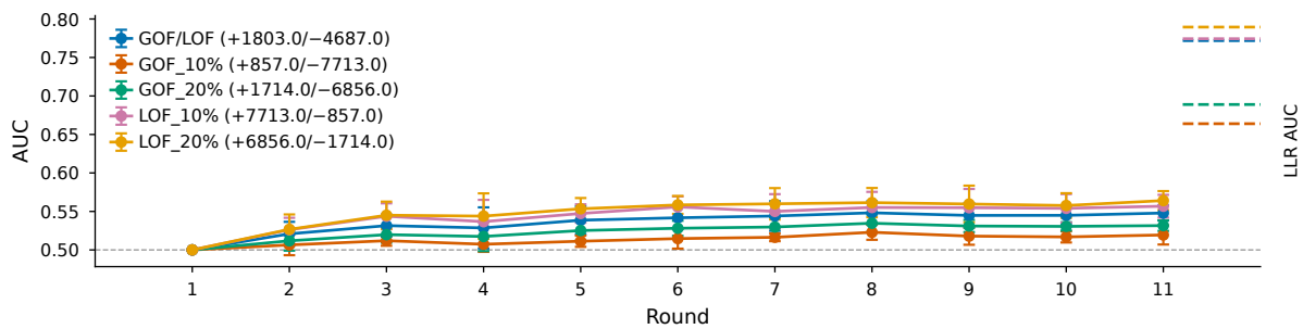
HXK4
