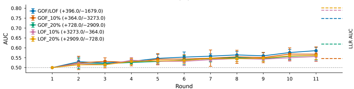
SRC
