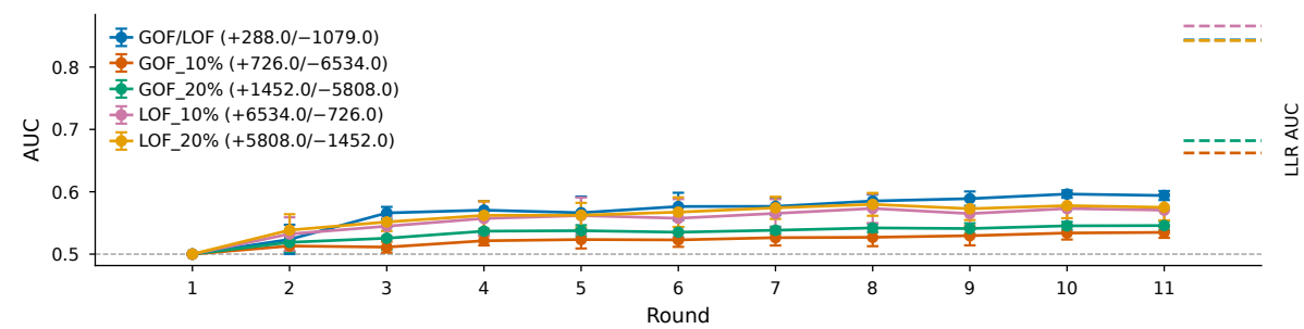
PTEN
