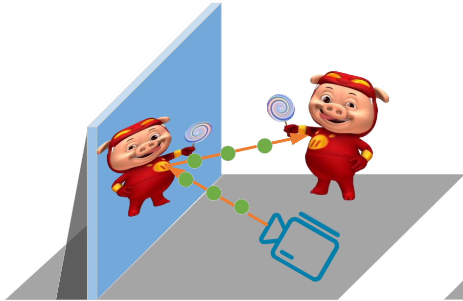
(a) Mirror-NeRF
