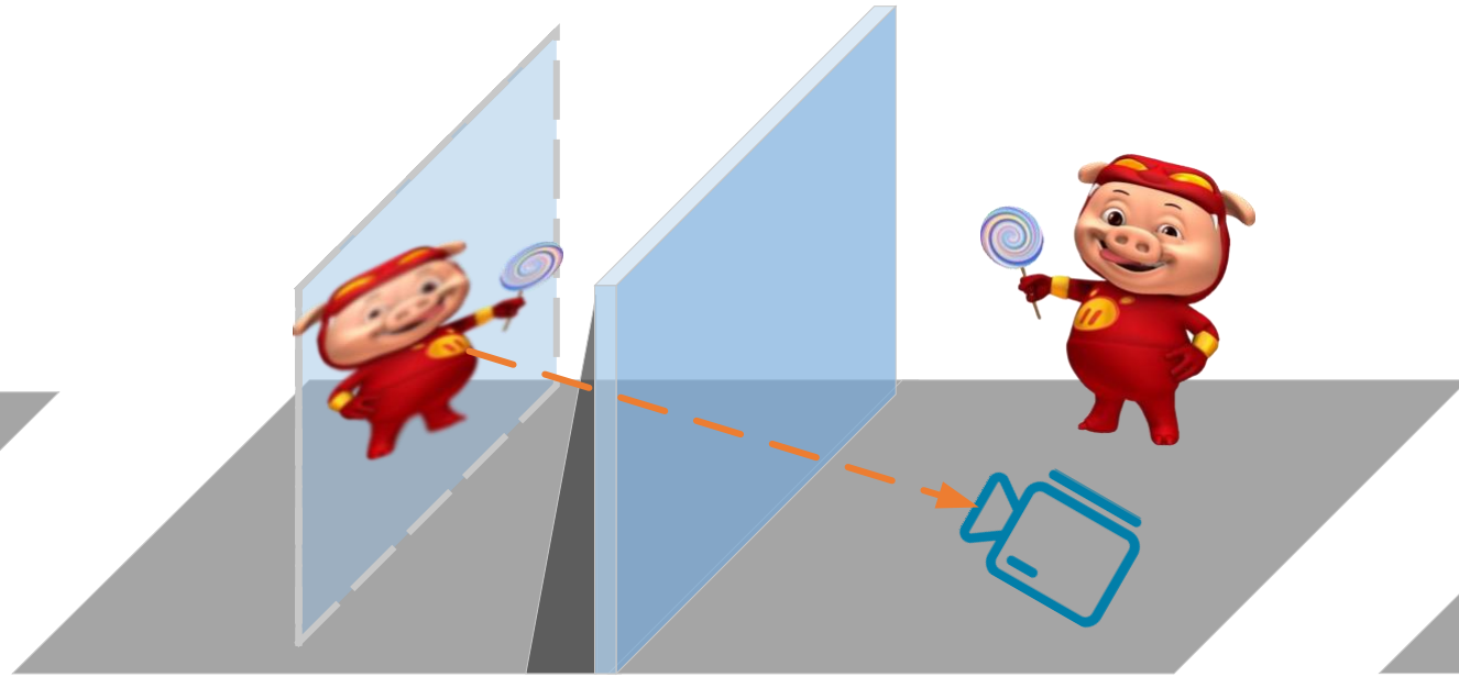
(b) 3DGS
