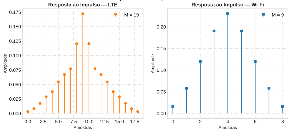
FIGURA 7 – Resposta ao impulso das máscaras
