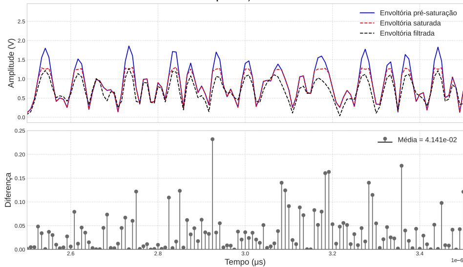
FIGURA 9 – Comparação das envoltórias e erro associado (antes da otimização plena).
