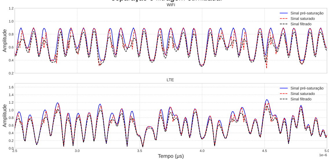
FIGURA 12 – Formas de onda individuais para os canais Wi-Fi e LTE após a separação e filtragem otimizada.
