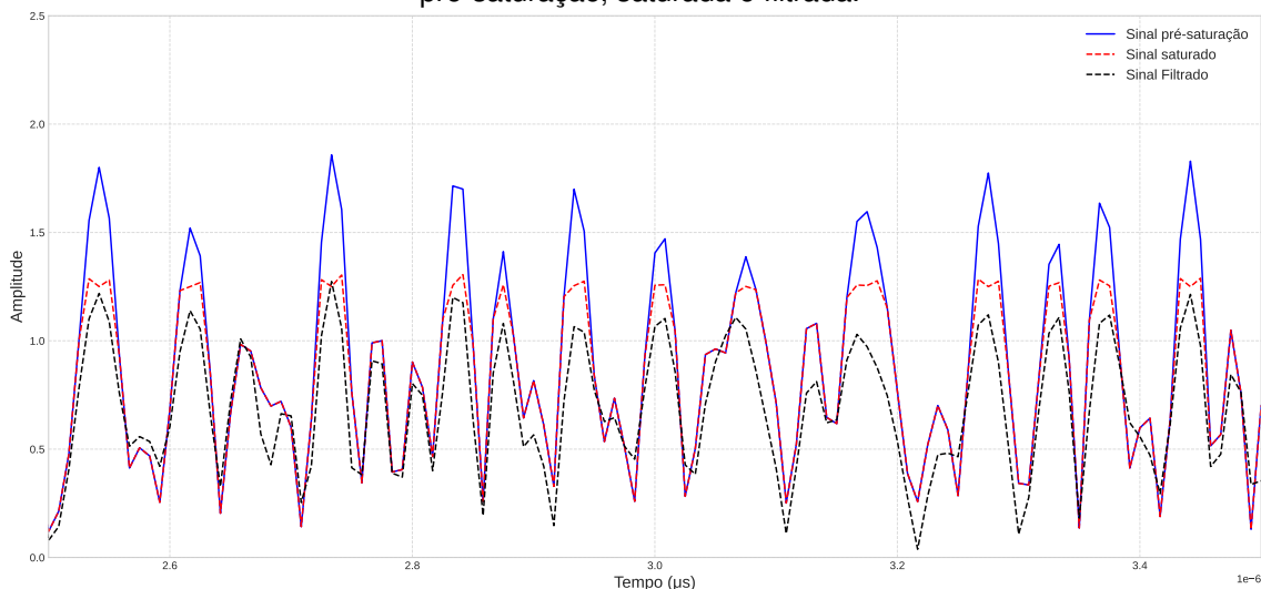
FIGURA 11 – Detalhamento do comportamento temporal das envoltórias pré-saturação, saturada e filtrada.
