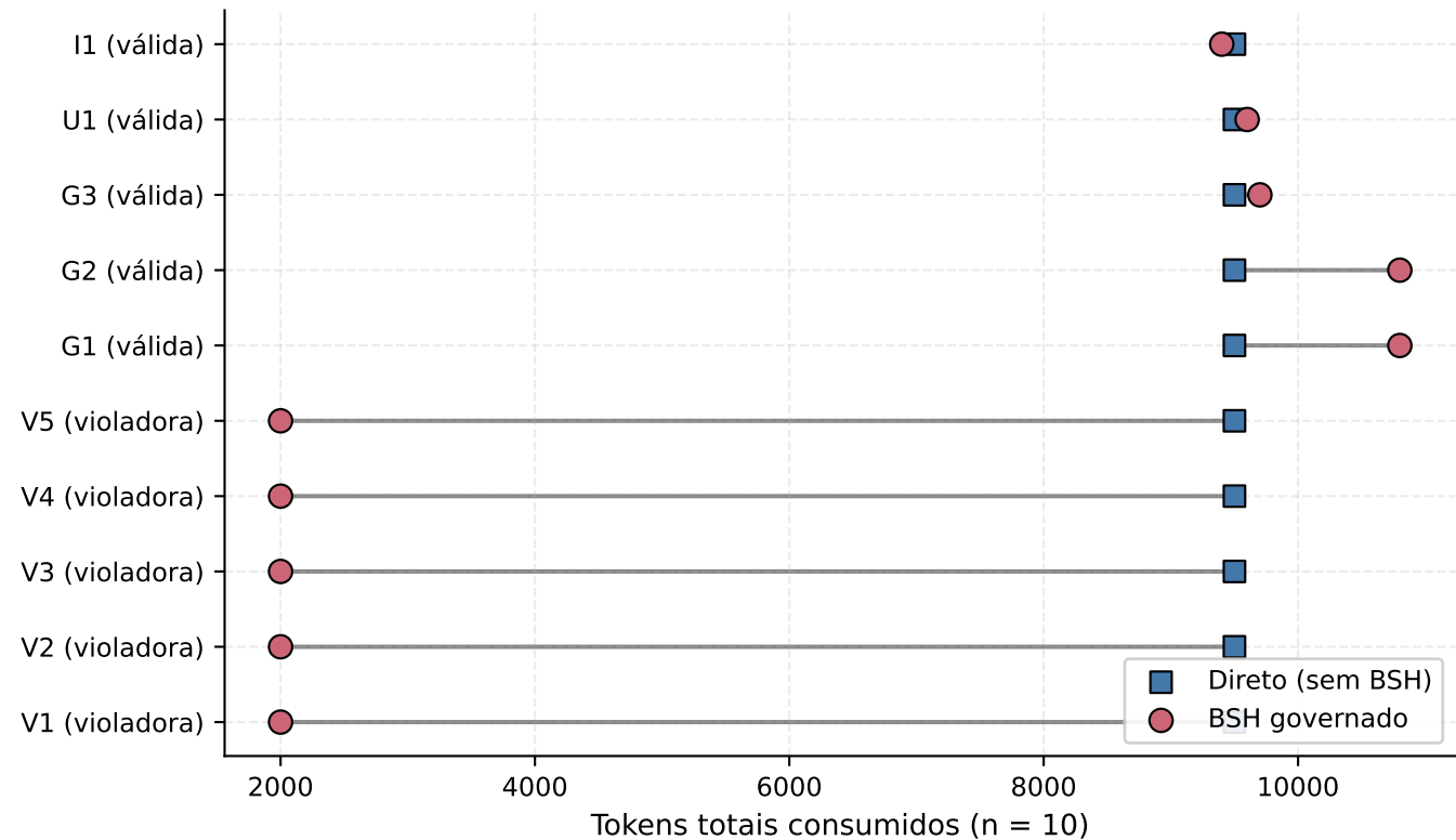
Consumo total de tokens pareado por tarefa (Dumbbell plot)
