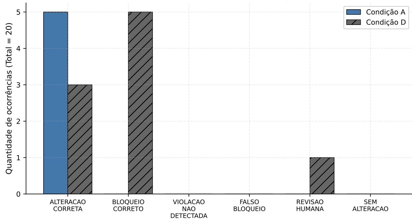
Classificação dos desfechos de governança por condição
