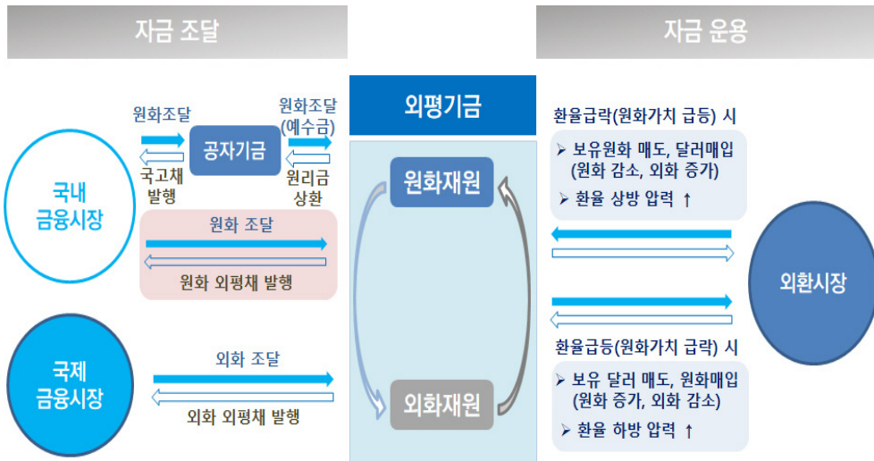
[외국환평형기금 개요]
